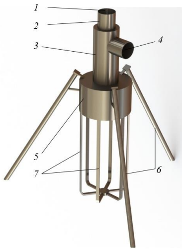
Рис. 1. Цифровой двойник классификатора с соосно расположенными трубами: 1 – входной патрубков, 2 – внутренняя цилиндрическая труба, 3 – внешняя цилиндрическая труба, 4 – выходной патрубков, 5 – цилиндрическая часть, 6 – опоры, 7 – металлическая конструкция для съемной емкости
